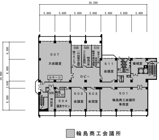
5階平面図
