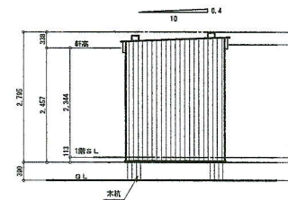
東側 立面図 S:1/100
