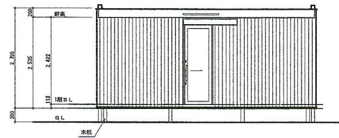
北側 立面図 S:1/100
