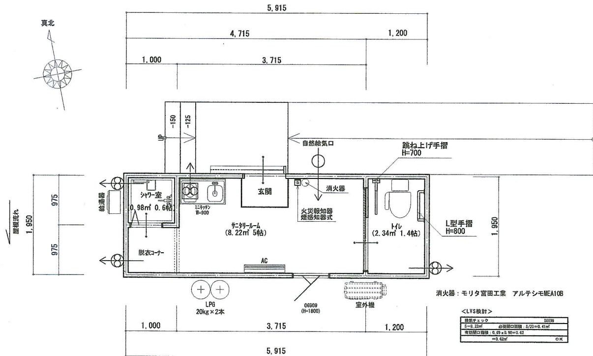
1階 平面図 S:1/50
