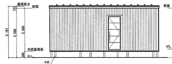
西側 立面図 S:1/100
