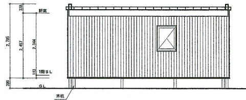
南側 立面図 S:1/100
