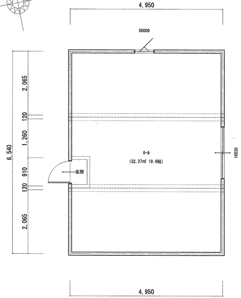
1階 平面図 S:1/50
