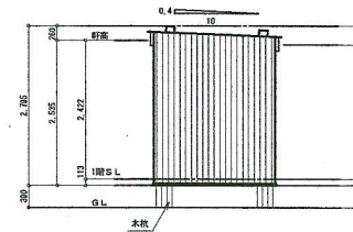
西側 立面図 S:1/100
