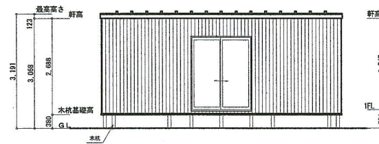
東側 立面図 S:1/100
