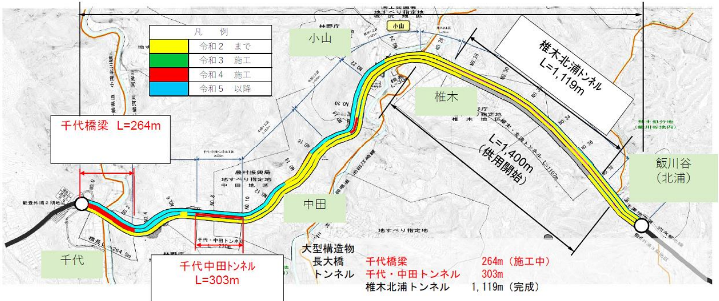
能登外浦4期地区 L=4.2km
